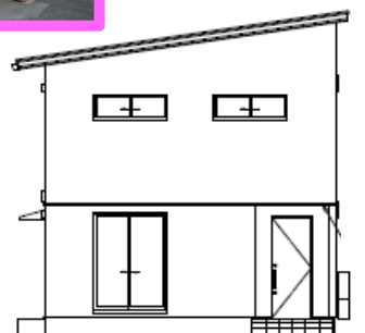
東側立面図
